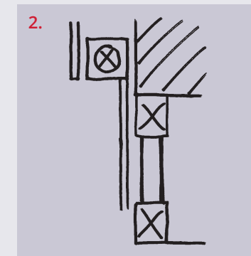
Verdunkelung außen verkleidet
