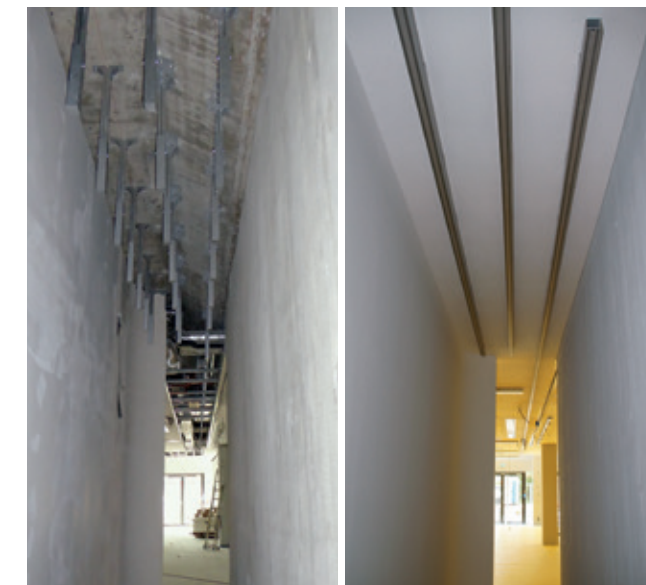
Parkraum Sprint-Vorhangschiene-Anlage in Aula
