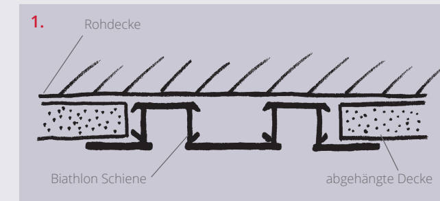
Biathlon integriert
