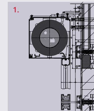
Sonnenschutz ZIP außen
