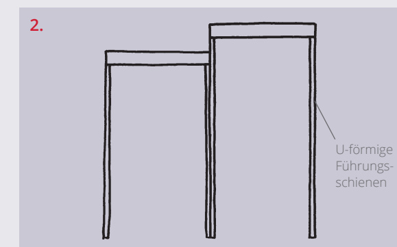
Rollo-Anlagen mit U-förmigen Führungsschienen, höhenversetzt
