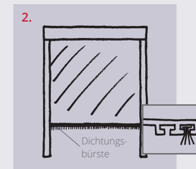
Rollo, Fallstab und Führungsschienen mit Dichtungsbürste
