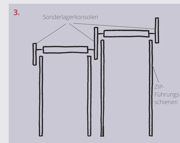
Offene ZIP-Anlagen, höhenversetzt
