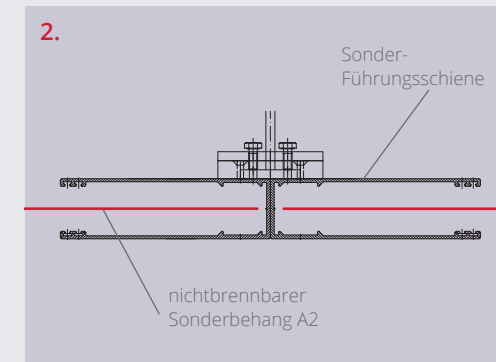
Schnitt Sonder-Führungsschiene mit Behang A2
