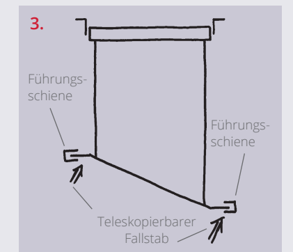
Fallstabgeführte Rollo-Anlage
