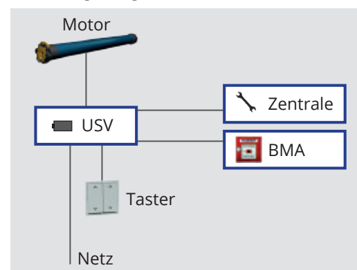
Notstromversorgung USV
