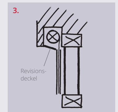
Voll integriert, revisionierbar
