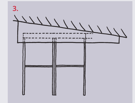
Offene ZIP-Anlagen mit Sonder-Verblendung
