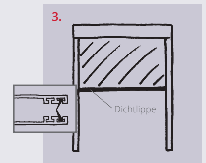
Rollo, Fallstab mit Gummidichtung
