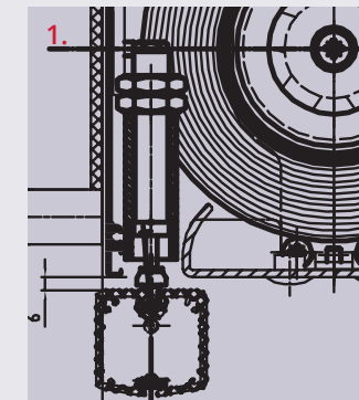
Rollo mit Standard-Fallstab
