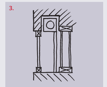
Rollo integriert im Zwischenfenster
