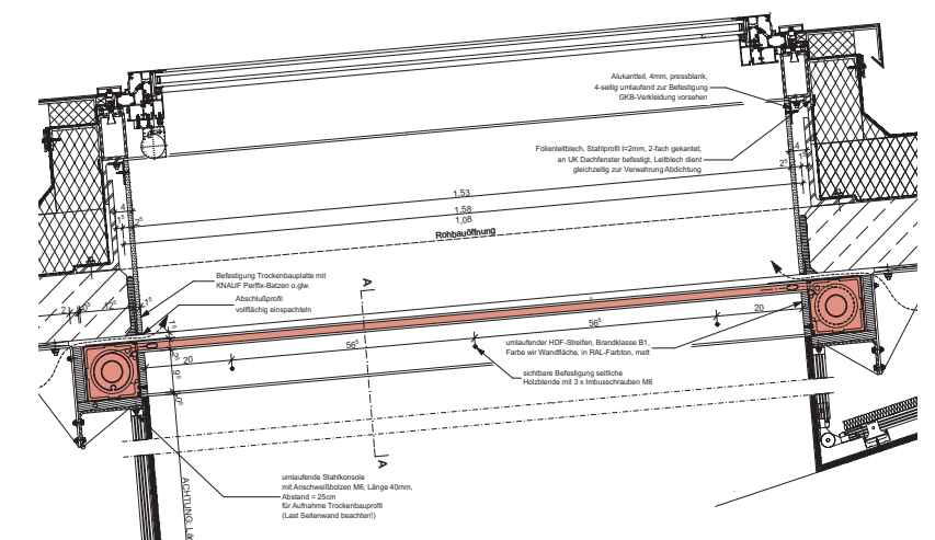
Rauchabzug Horizontale ELS-Anlage
