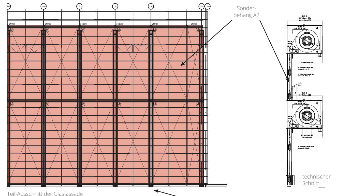
Teil-Ausschnitt der Glasfassade
