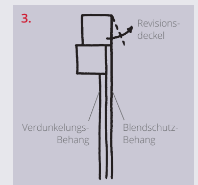
Gehäuse übereinander revisionierbar
