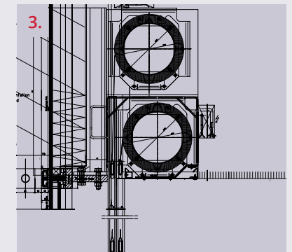
ZIP Verdunkelungsanlagen innen
