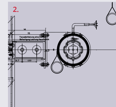
Blendschutz innen
