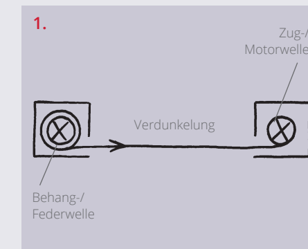
Einzelanlage – nur Verdunkelung
