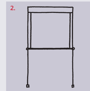
Seilgeführte Rollo-Anlage
