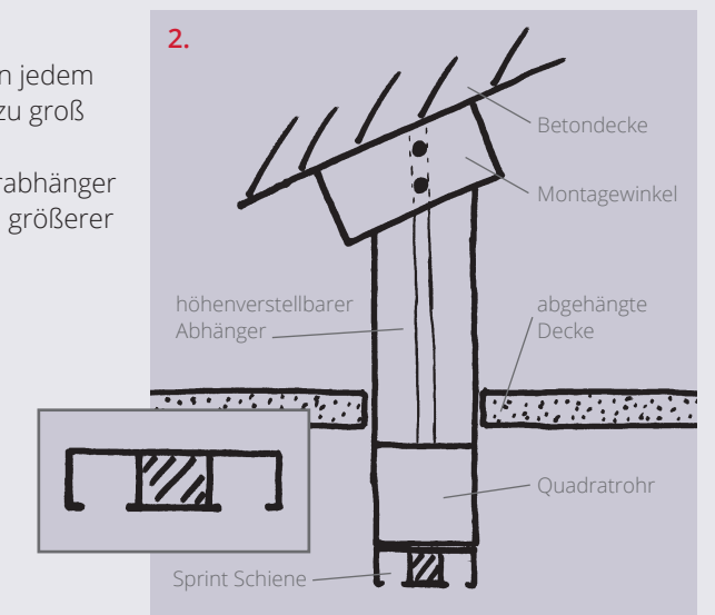
Sprint inkl. Sonderabhänger u. abgehängter Decke
