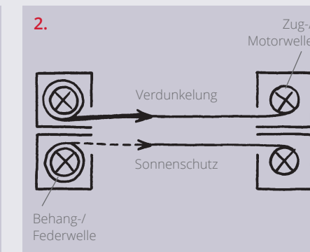
Zwei übereinanderliegende Einzelanlagen
