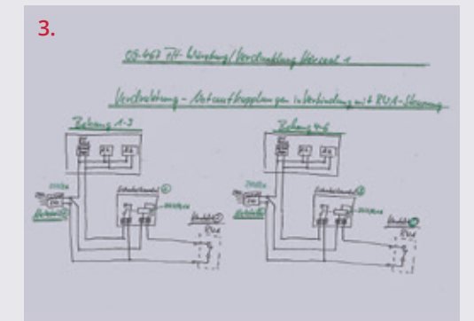
Schema-Steuerung Not-Auf
