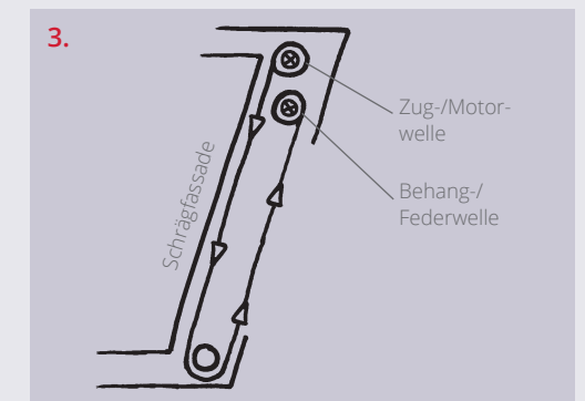
Vertikale Gegenzuganlage
