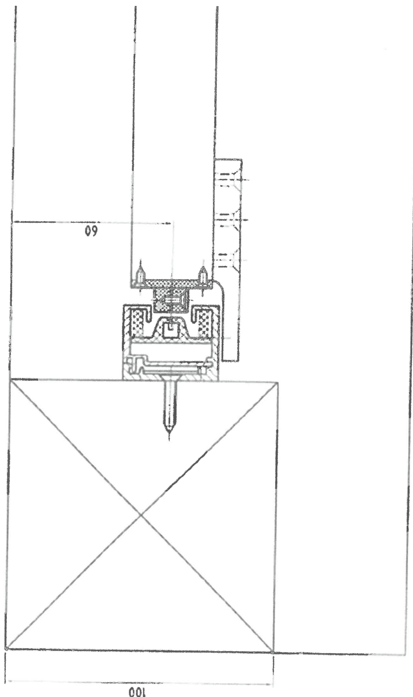
Bild 3 Technische Zeichnung: „Brichta Blend-, Sonnenschutz- und Verdunklungssystem ZIP Modell: BS-ZIP-MQ3“
