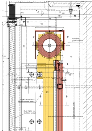
Bild 2: Technikumsetzung
